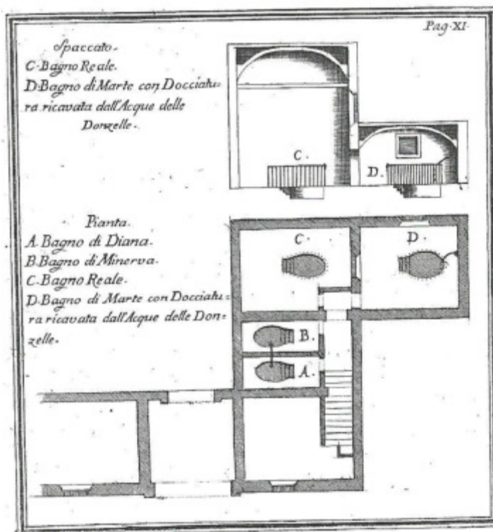
Disegno e pianta del bagni Reale, Marte, Diana e Minerva dal trattato del Bassi.
